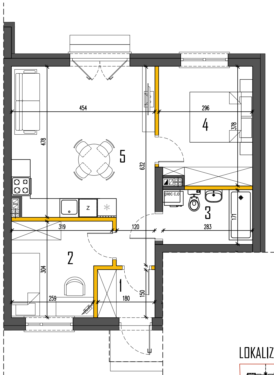
RZUT PARTERU
