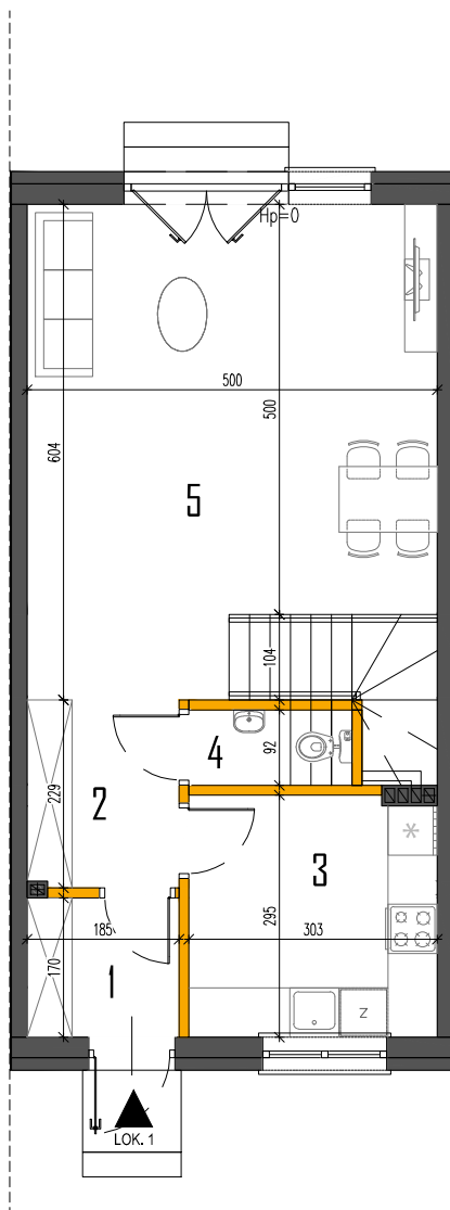
RZUT PARTERU
