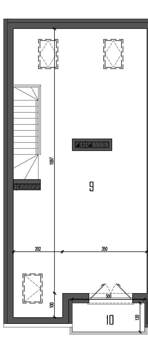
RZUT PODDASZA
