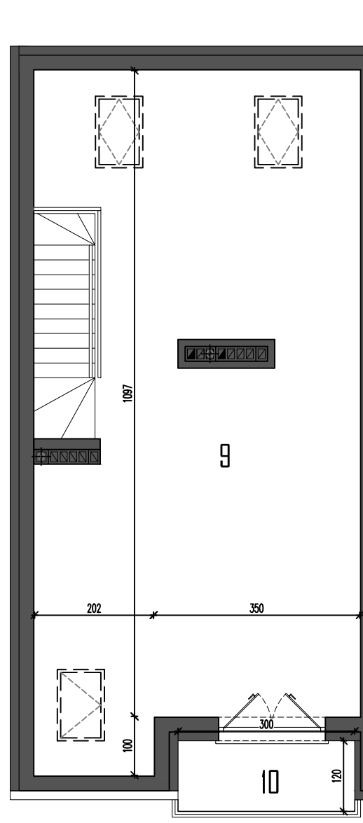
RZUT PODDASZA
