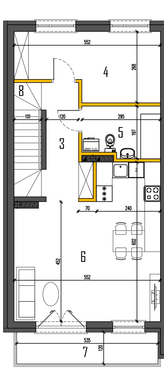
RZUT PIĘTRA
