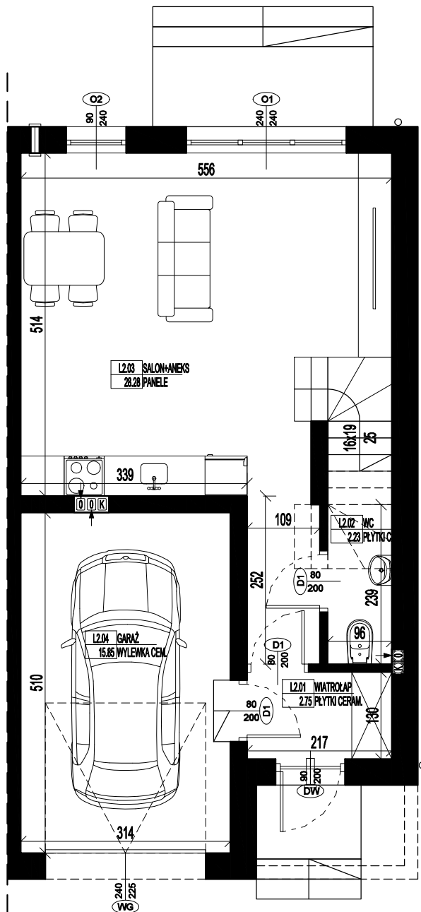
RZUT PARTERU LOKAL 2
