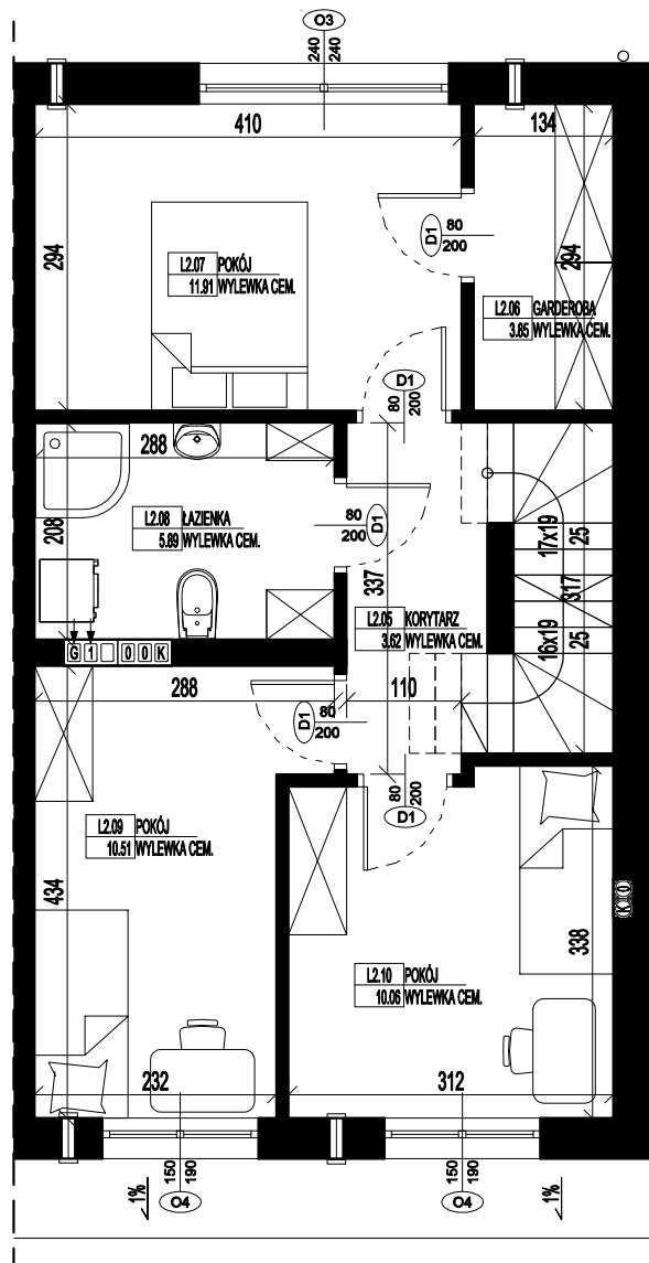
RZUT PIĘTRA LOKAL 2
