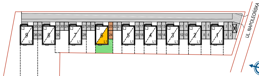
RZUT PARTERU
