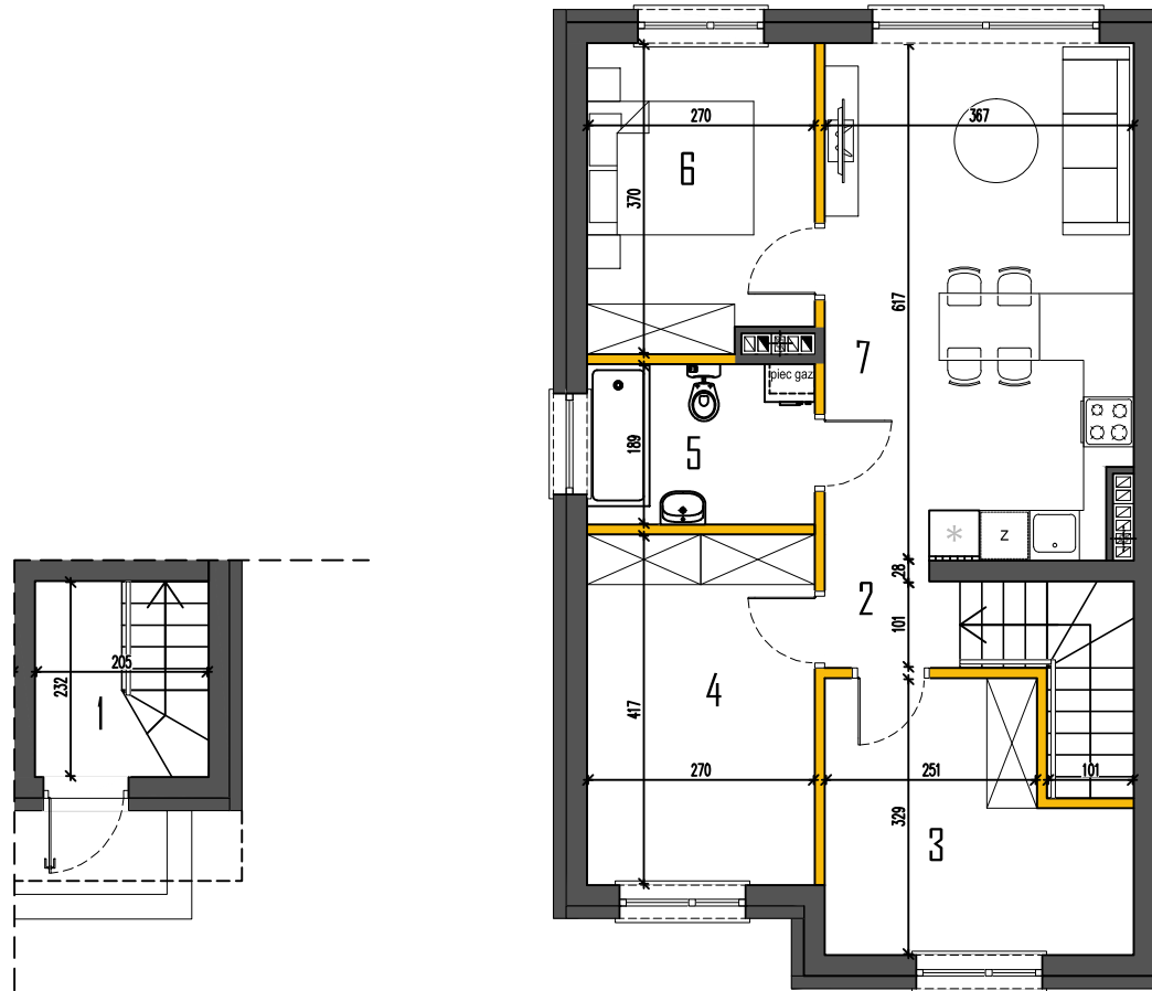
RZUT PARTERU
