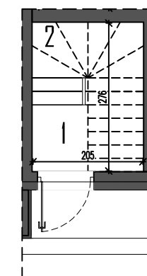
RZUT PARTERU
