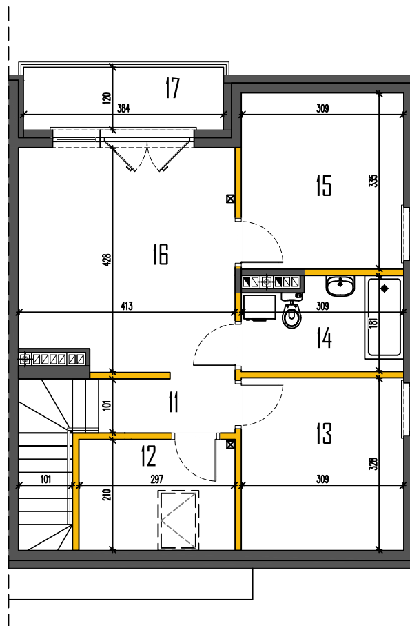
RZUT PODDASZA
